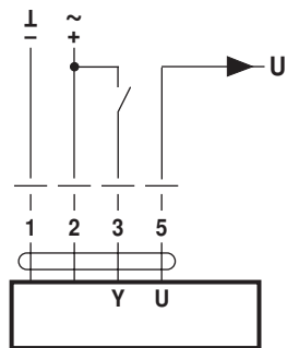
Sterowanie Zamknij/Otwórz
